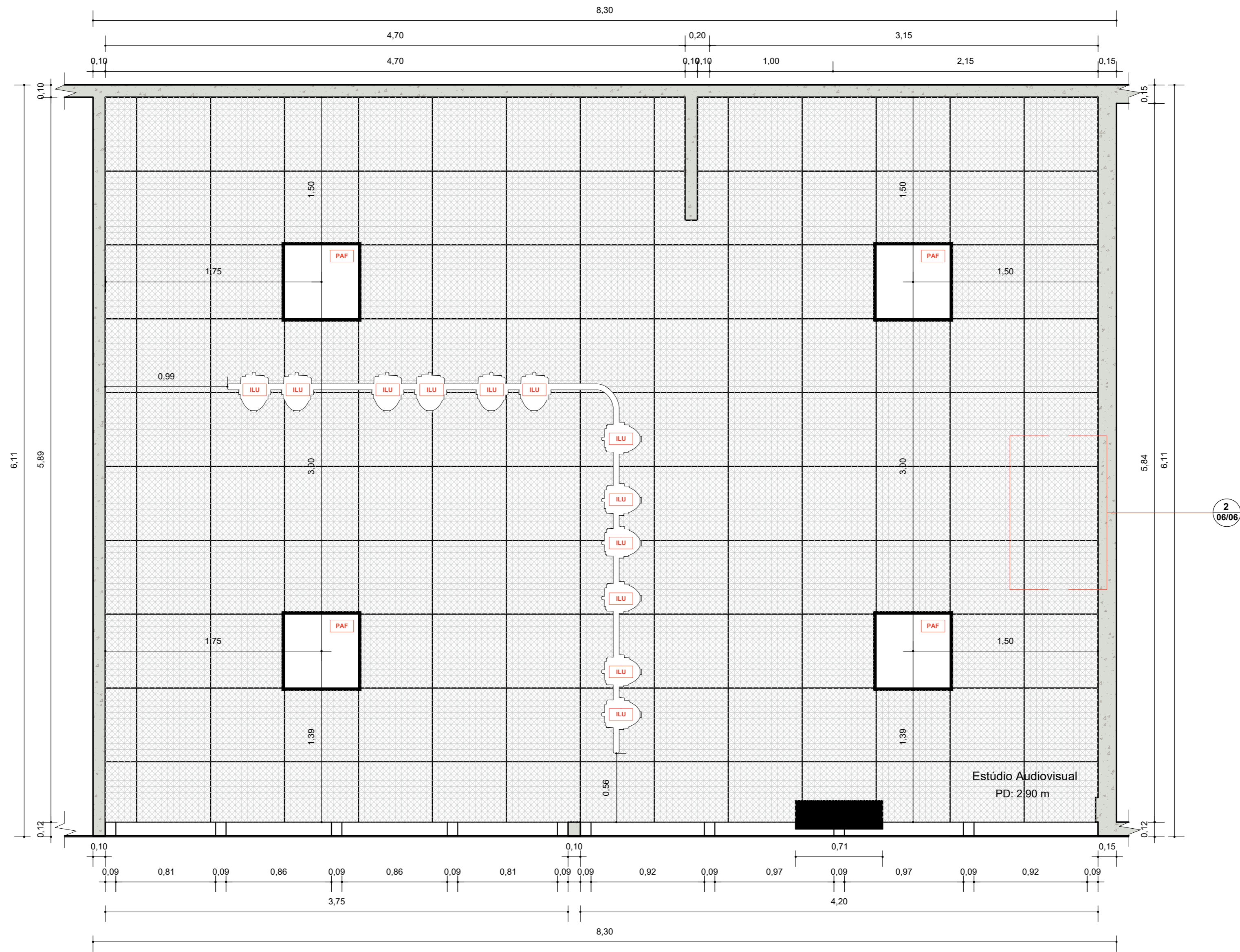
5 PLANTA BAIXA - FORRO ESCALA 1:25
